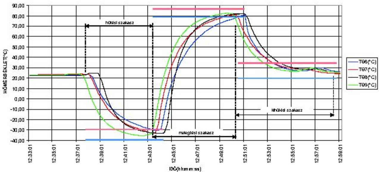
Hideg-meleg alagút hőmérséklet eloszlás
