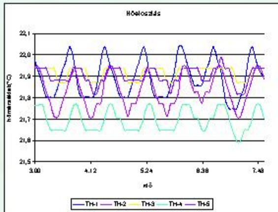
Hideg-meleg alagút hőmérséklet eloszlás
